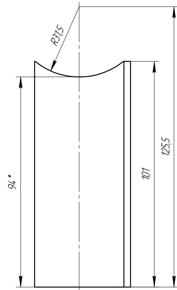
Дет. поз. 2
