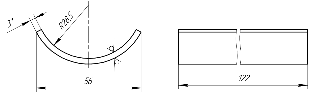
Дет. поз. 3
