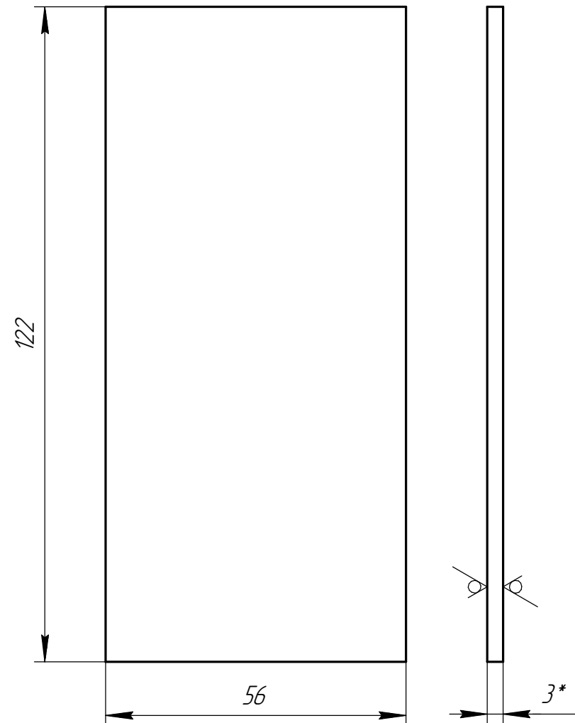
Дет. поз. 1
